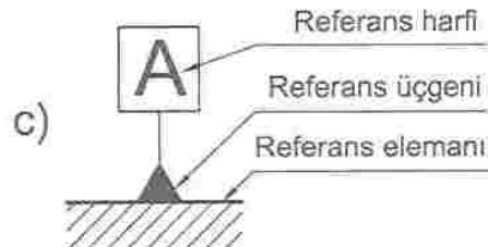
Şekil 52: Çerçeve elemanları
