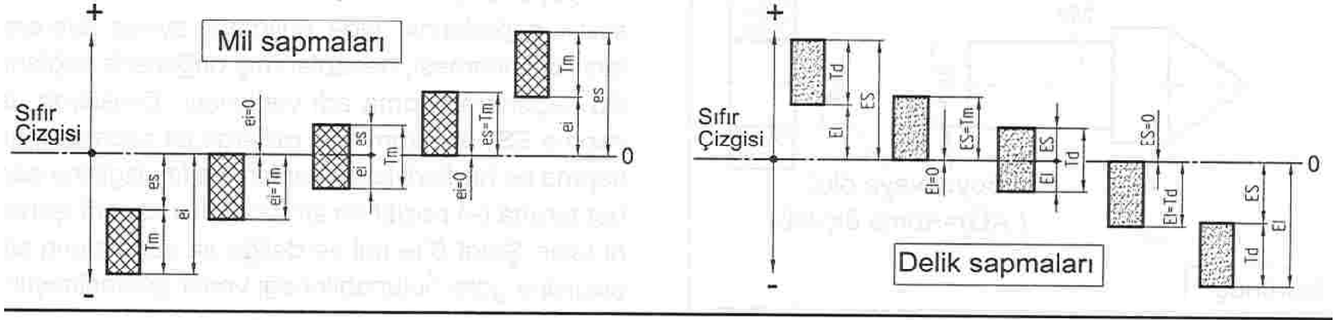
Şekil 5: Mil ve deliklerde sapmalar
