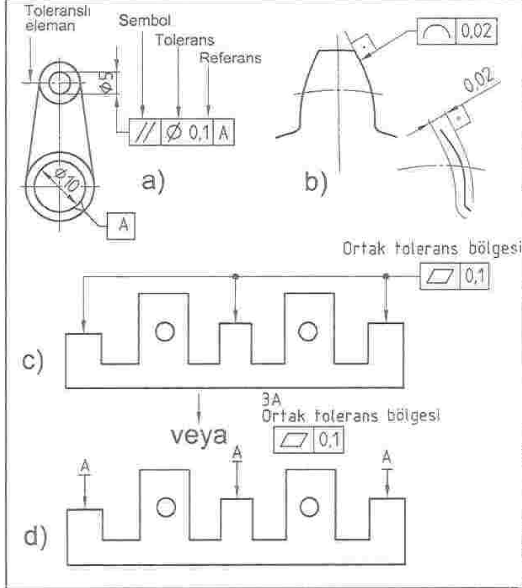
Şekil 53: Tolerans bölgelerinin gösterilmesi
